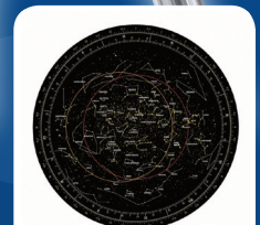
Sternkarte/Star map
